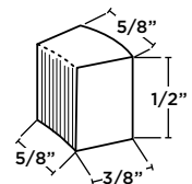
Cubelet Dimensions
